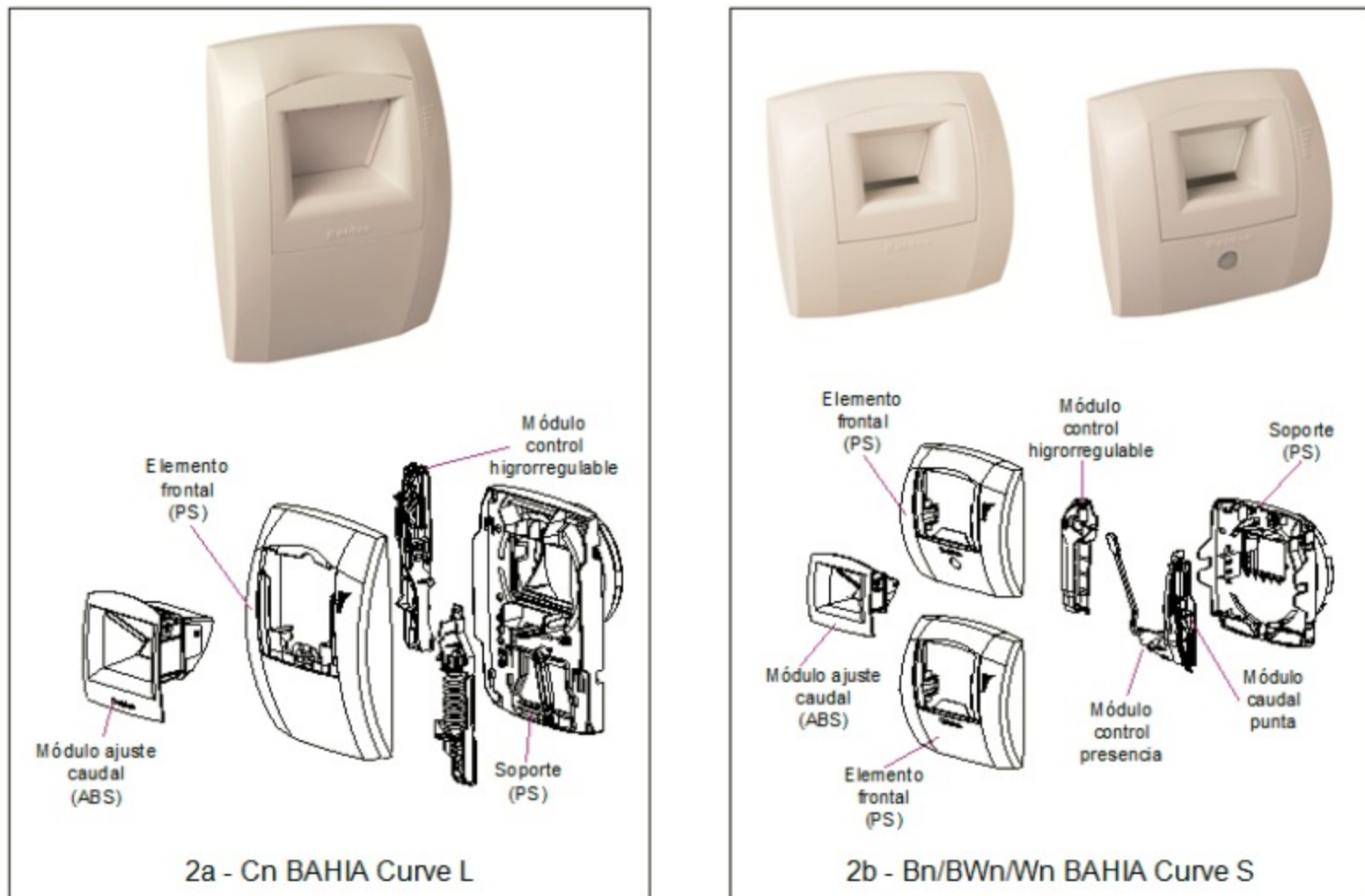
Figura 2. Bocas de extracción
